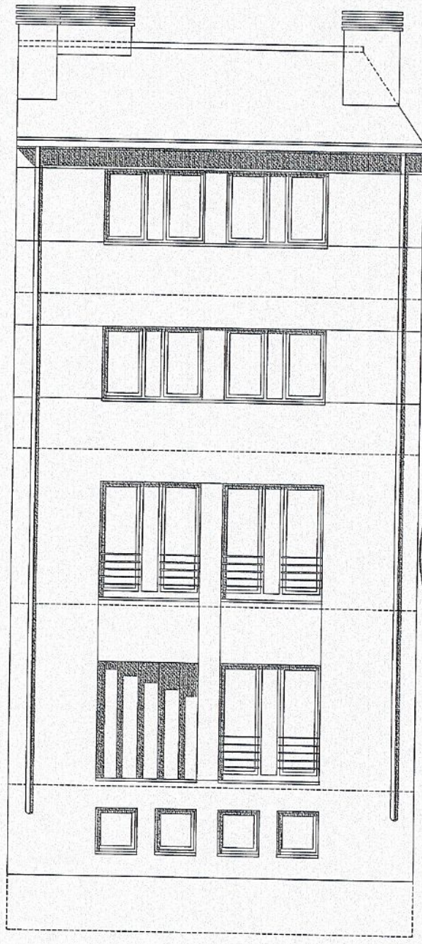
ALZADO A PATIO
