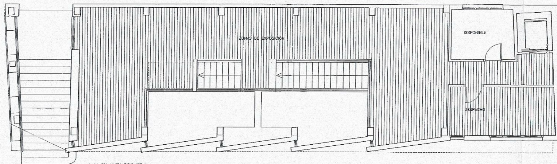
ENTREPLANTA PRIMERA 109,70 m2
