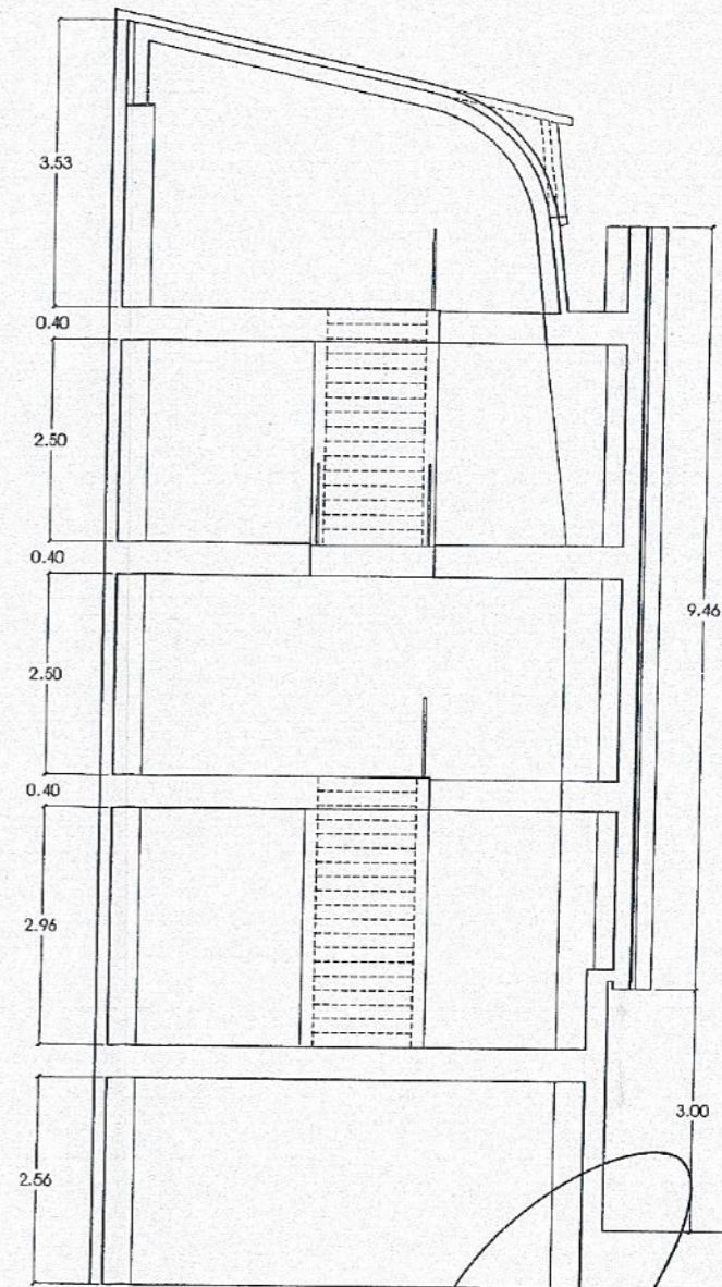
SECCIÓN TRANSVERSAL
